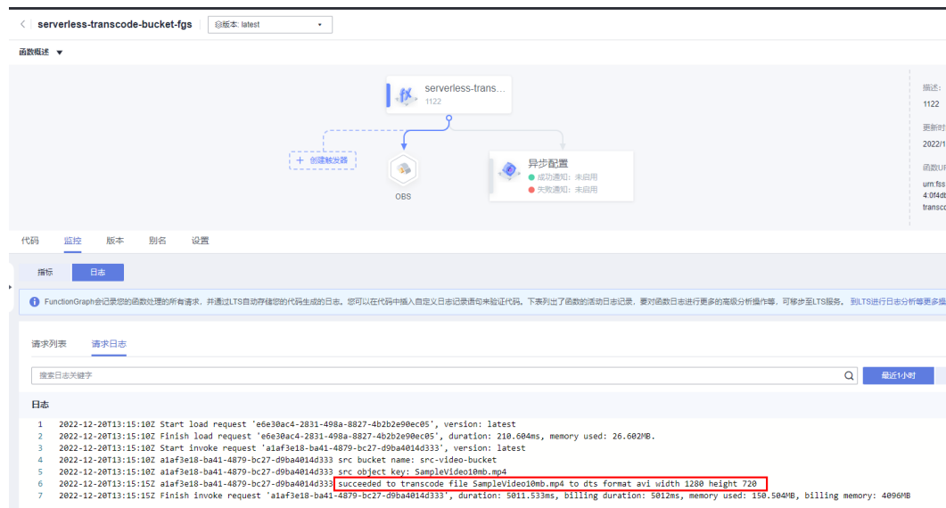
图5 请求日志
